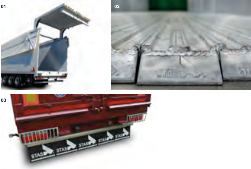
01 Zweiteiliges Dachnetz mit hydraulischer Tür 02 HDI Bodenbretter 03 Rückleuchtenabdeckung
